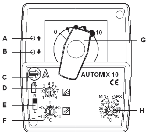
Kuva 2. Säätömoottorin etupinta.
